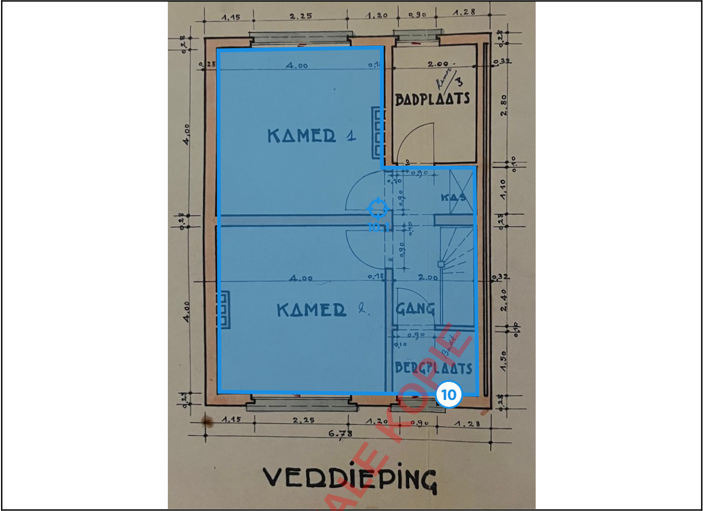
Legende van plan 1.3: 1ste verdiep
