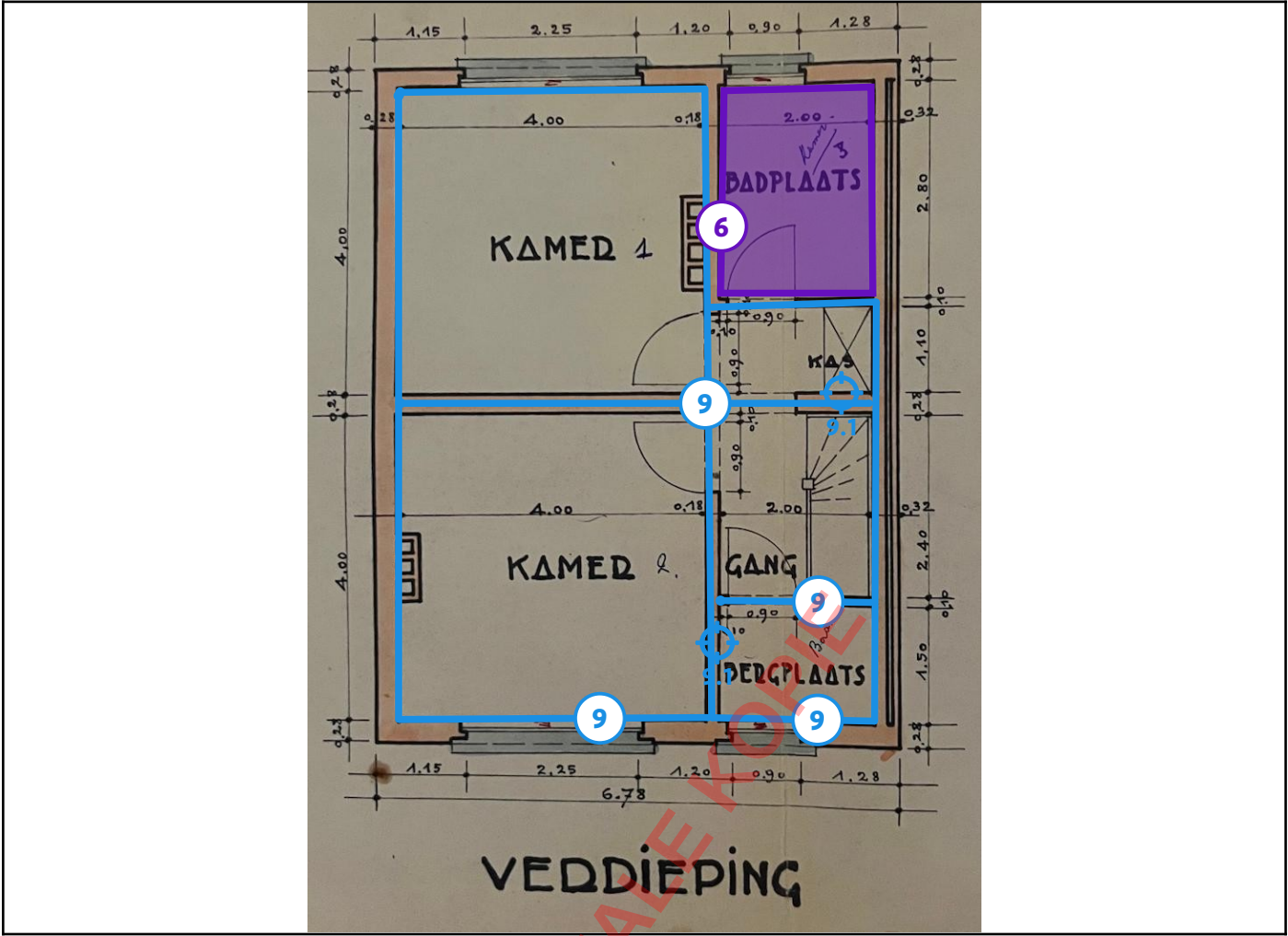
Legende van plan 1.8: 1ste verdiep
